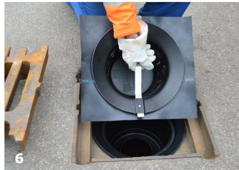
coalsi® Filterrahmen mit Dichtung einsetzen
